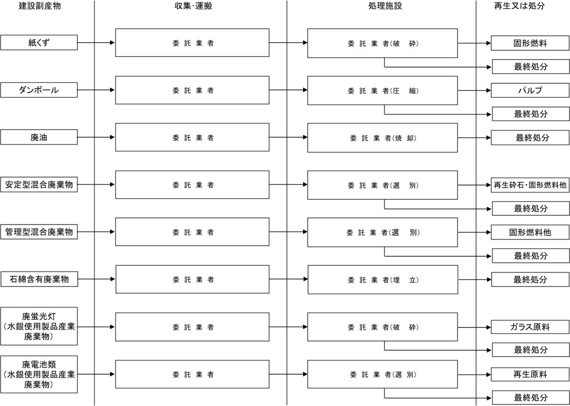
別紙1-2 産業廃棄物の一連の処理の工程
