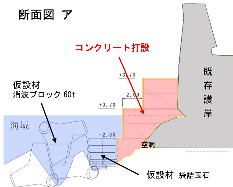
断面図 イ
