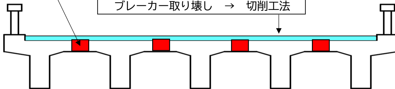
既設橋 断面
