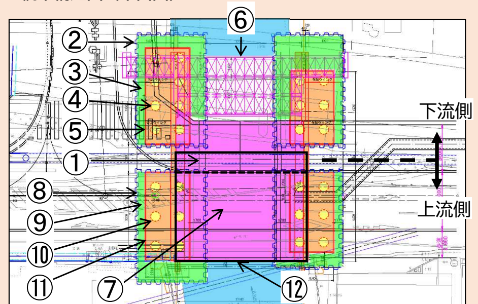
橋梁構造図（平面図）
