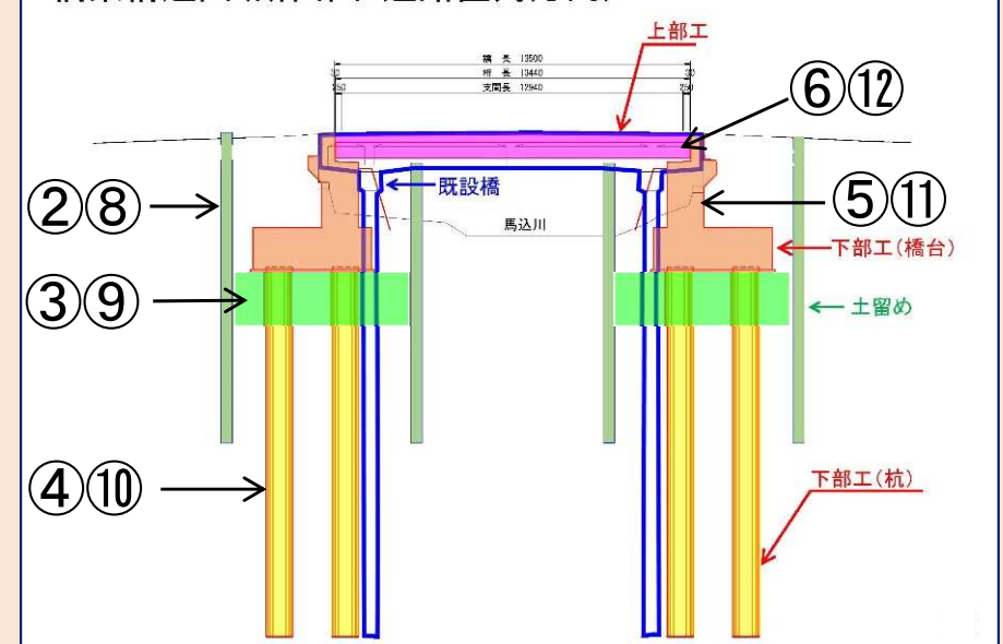
橋梁構造図（断面図・道路直角方向）
