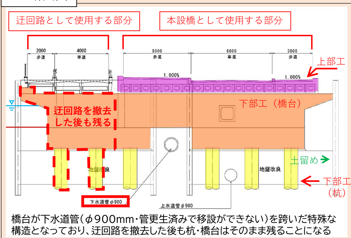
a-a'断面図
