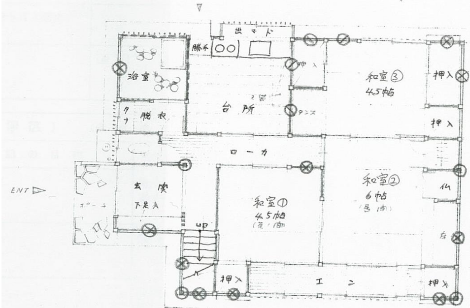
1階間取図
