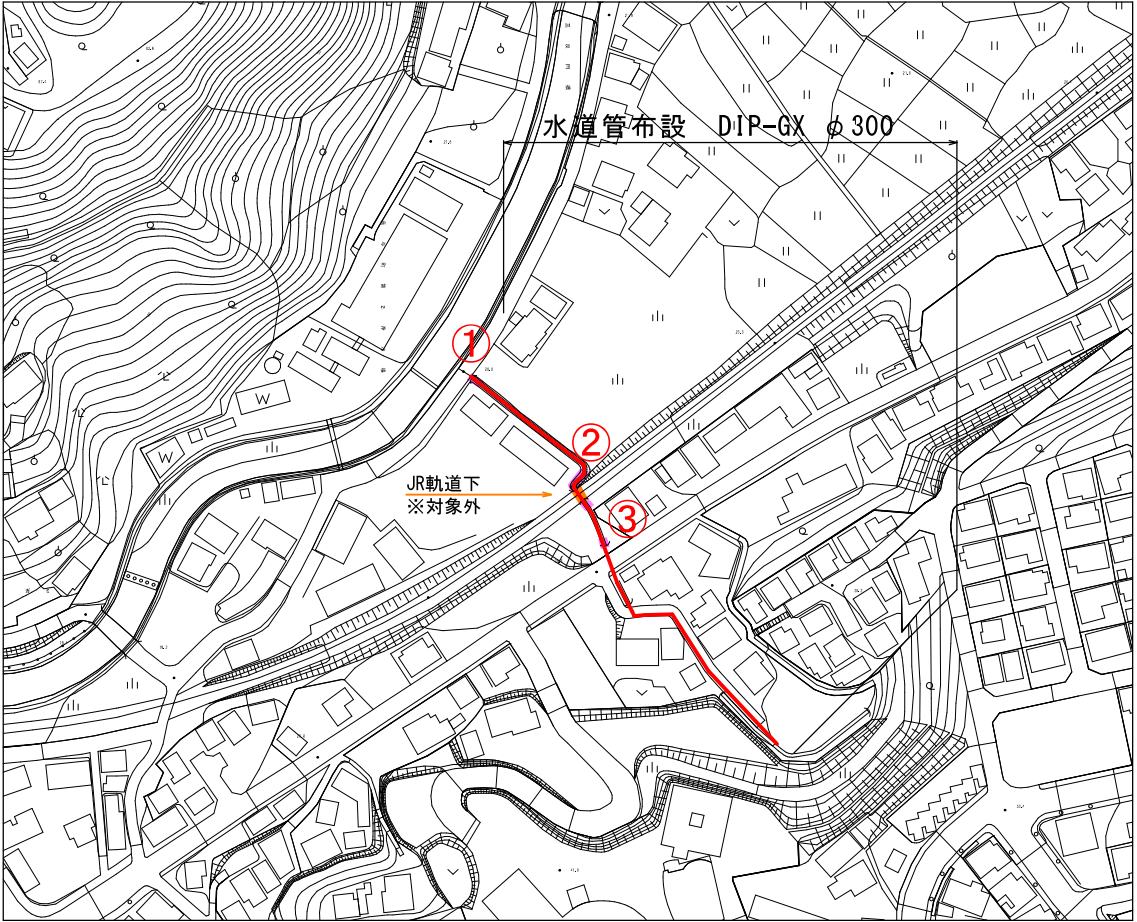
水路平面図 S=1:1000
