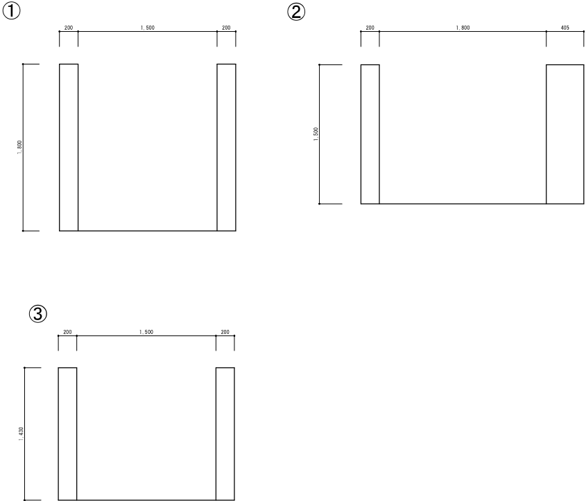
水路断面図 S=1:20
