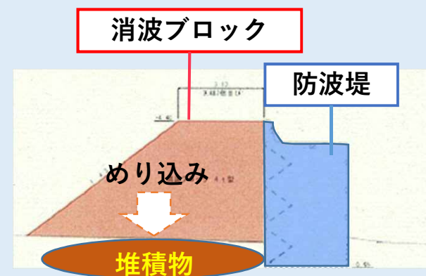
【図7 断面イメージ】
