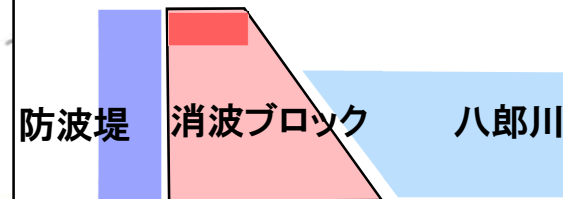
上流側より見た断面
