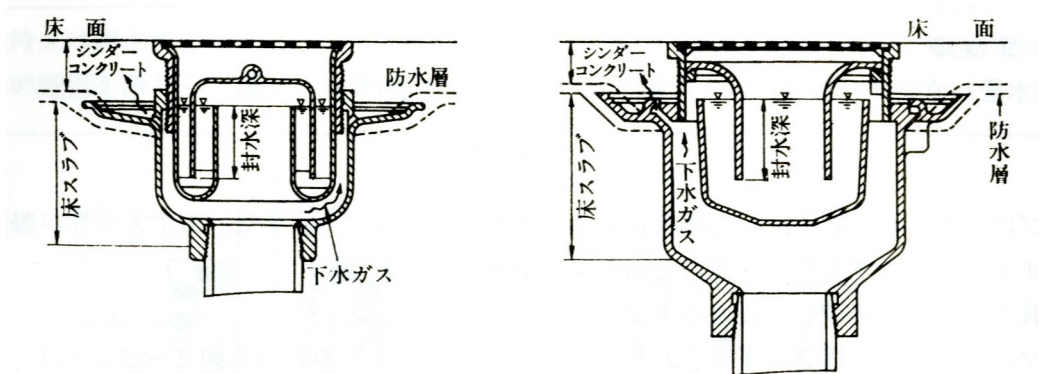
図 2-7 望ましくないトラップの例
