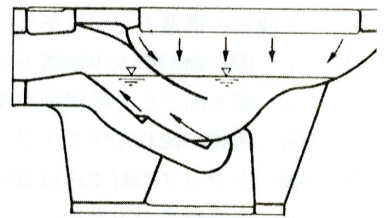
図 2-20 ブローアウト式
