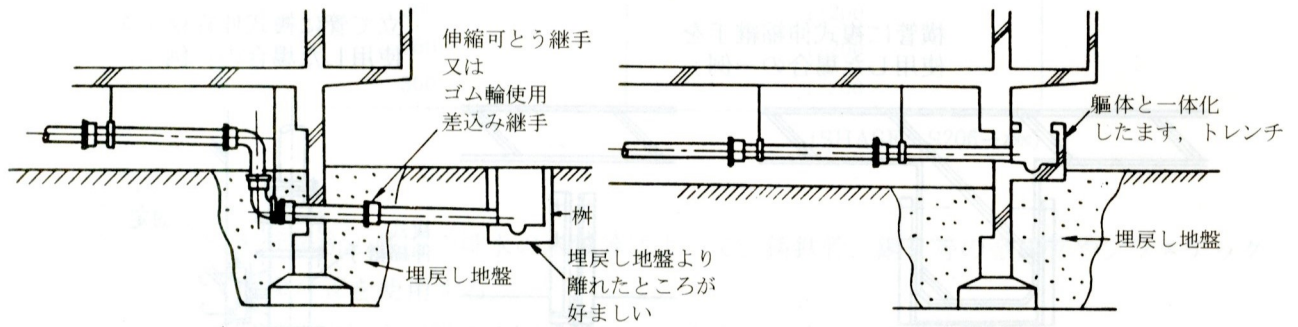
図 2-5 排水管・ますの地盤沈下変位に対する対策の例
