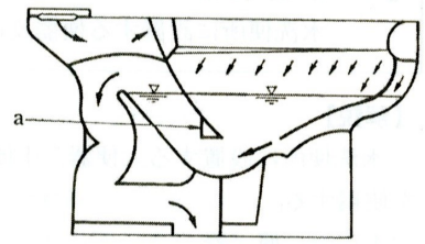
図 2-19 サイホンゼット式
