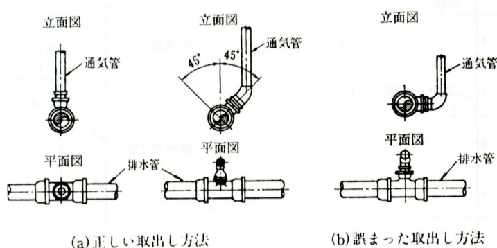
図 2-36 通気管の取出し方法
