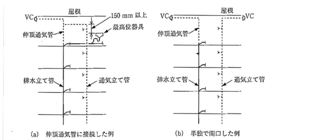
図 2－3 4 通気立て管の上部の処置
