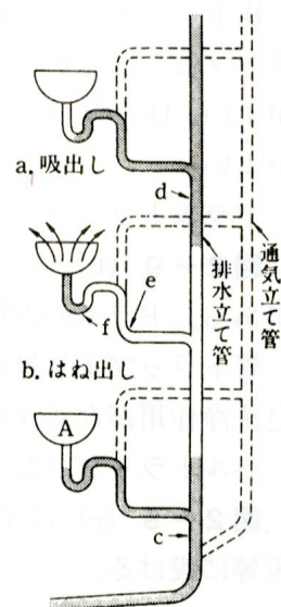
図 2-11 吸出し作用とはね出し作用
