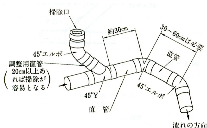
図 3 - 1 0 排水管の屈曲点でますが設置できない場合の掃除口と配管の例
