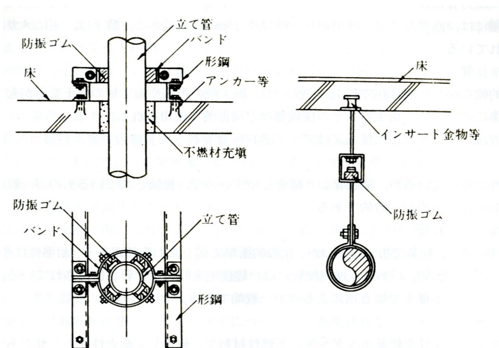
図 2-4 振動を考慮した管支持方法の例
