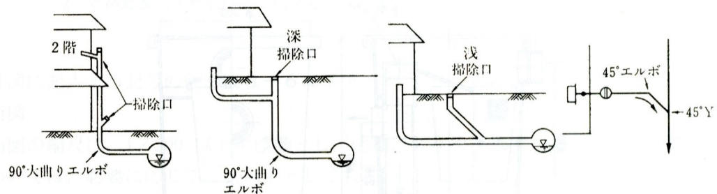
図3-9 会合点にますが設置できない例
