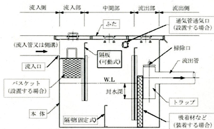
図6－1 阻集器の構造各部の名称
