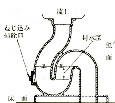
図2-8 ネジ込み掃除口の例
