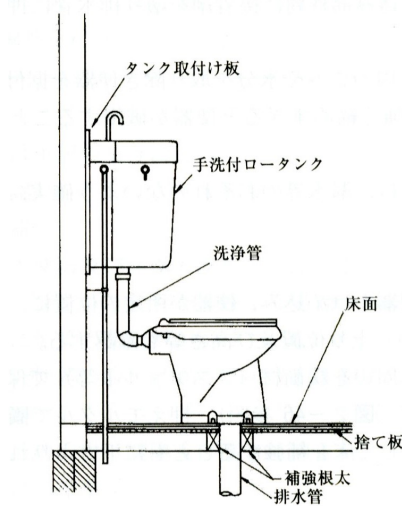
図 2-43 洋風大便器の施工例（ロータンク式）
