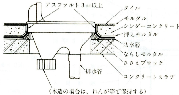
図2-44 和風大便器の施工例
