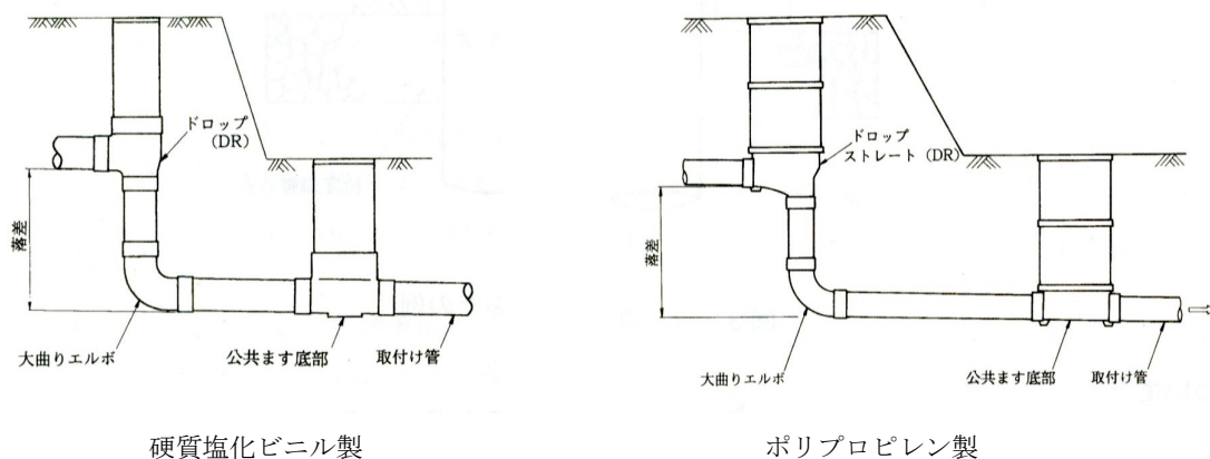
図3-6 (参考) 特殊ます (プラスチック製) の例
