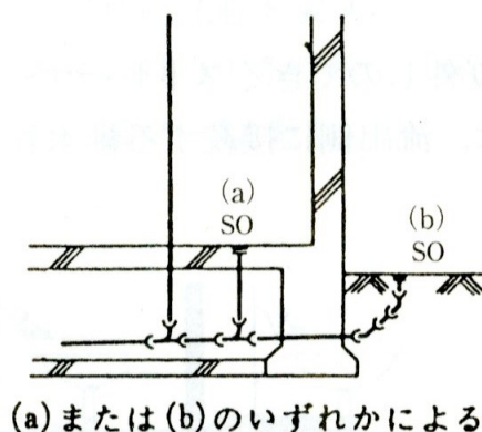
図 2 - 1 5 掃除口の取り付け状態の例
