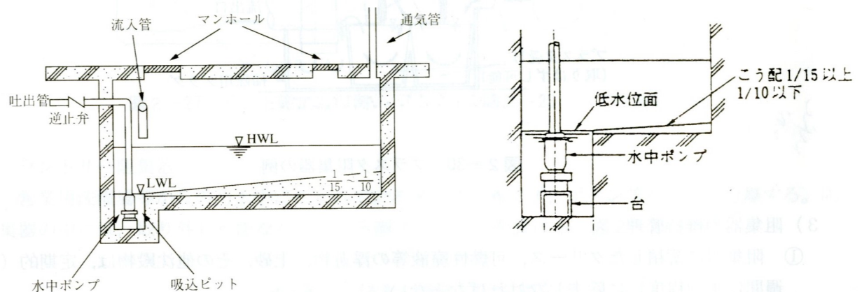
図 2-30 排水槽の例
