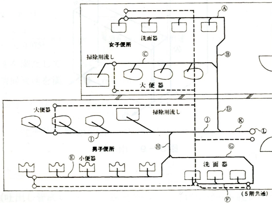
図9-2 各階系統図
