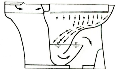
図2-17 洗落し式
