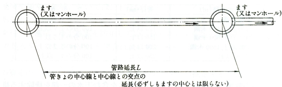
図 3-1 管路延長
