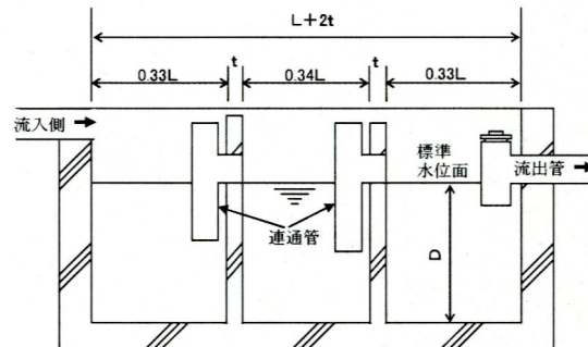
図 6-3 3 槽式独立槽形阻集器の隔壁の設置位置
