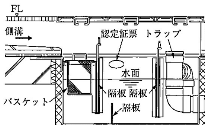
図 2-24 グリース阻集器の例
