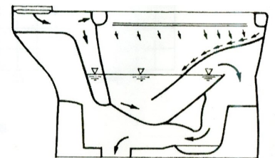
図2-18 サイホン式
