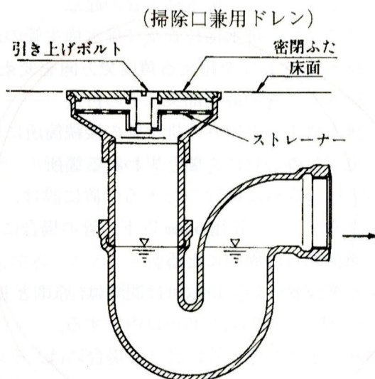
図 2-13 床排水トラップの例
