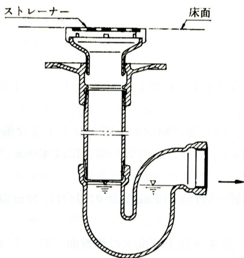
図 2-12 床排水トラップの例
