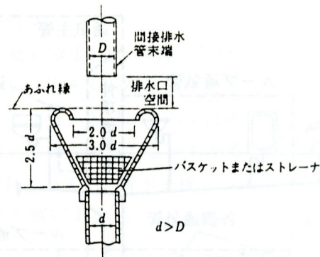
図 2-3 2 排水口空間
