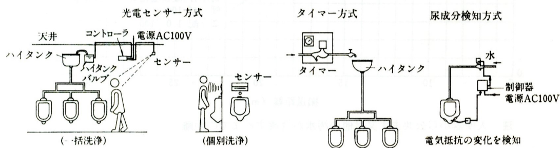
図 2-23 小便器の節水方式
