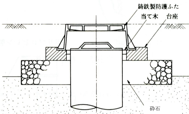
図3-4 小口径ますの保護
