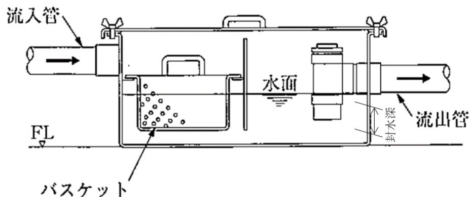
図 2-29 プラスタ阻集器の例
