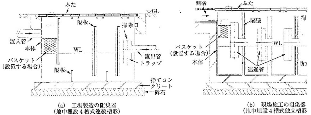
図 2-25 オイル阻集器の例
