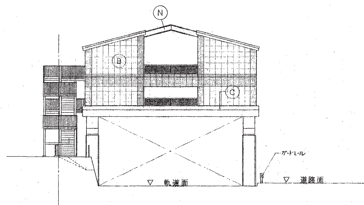
西 立面図 1:200
