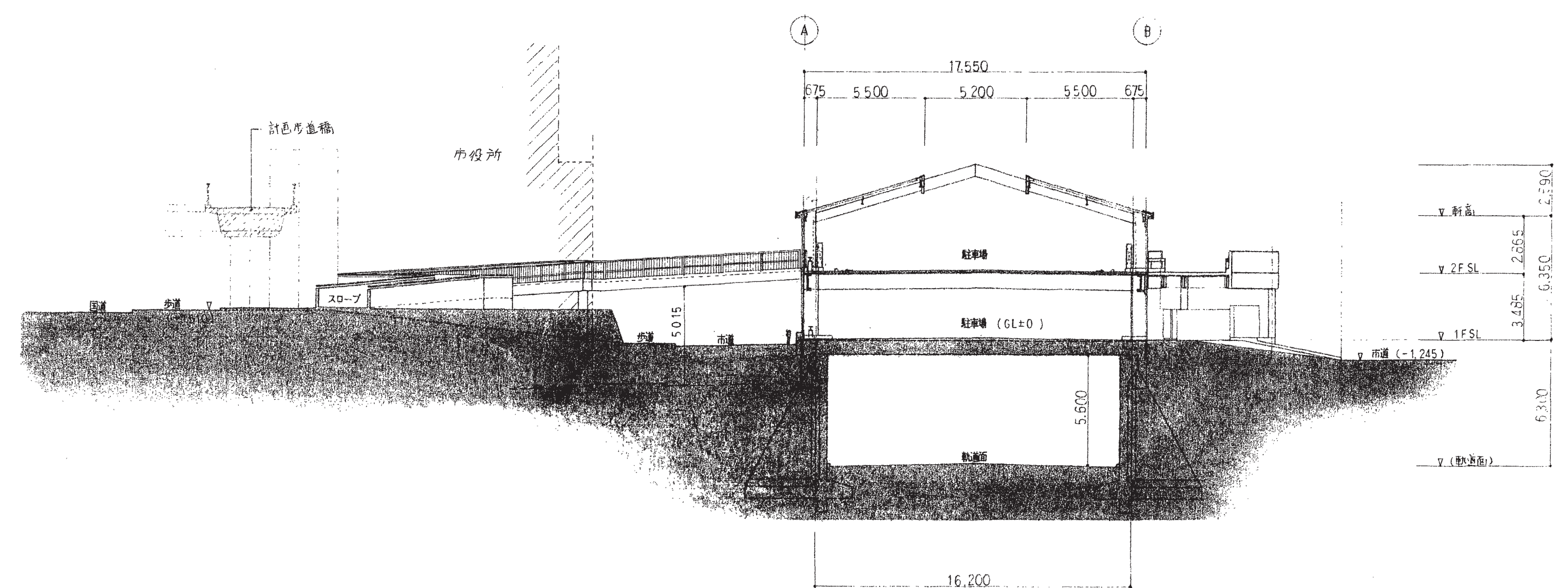
12通り 断面図 1:200
