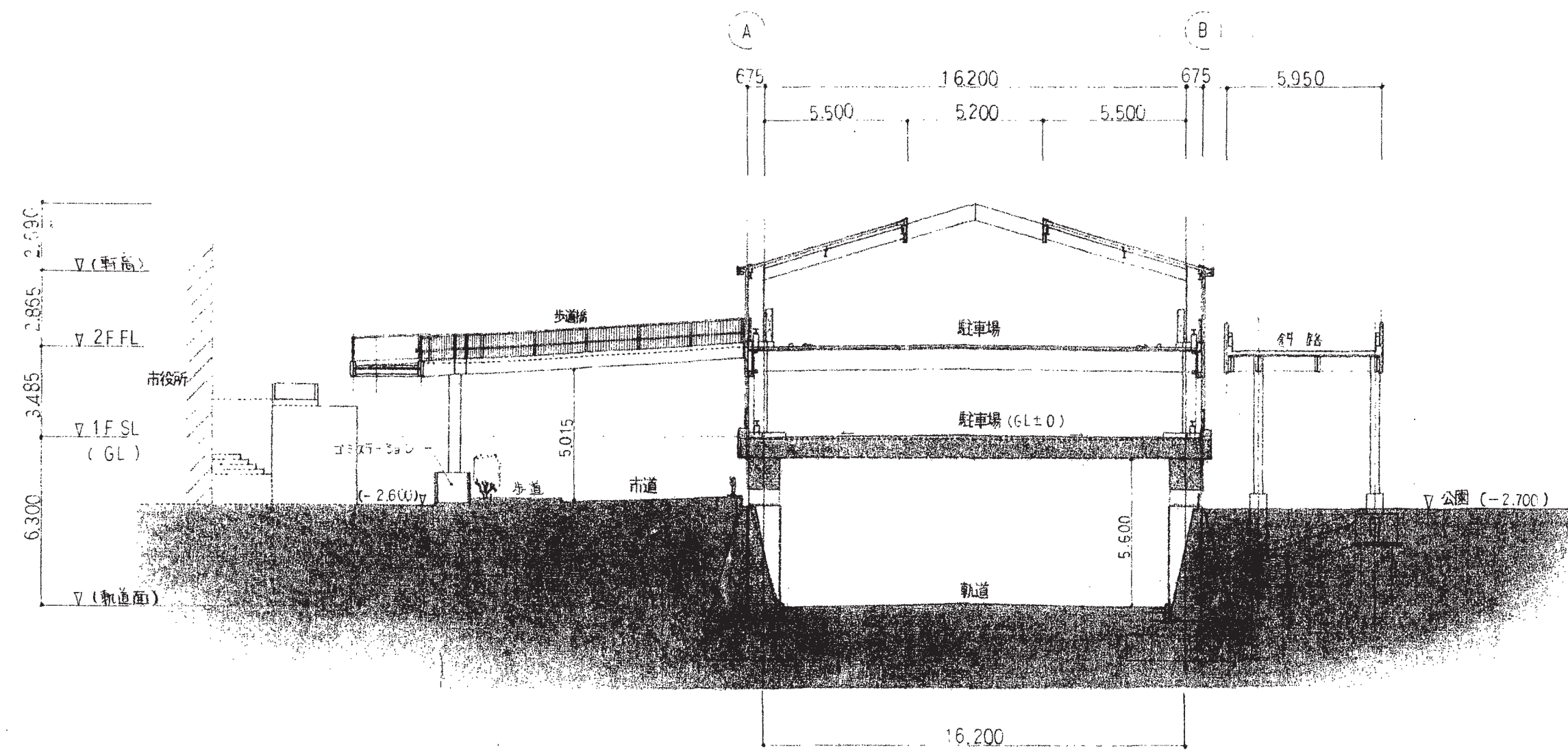
10通り 断面図 1:200
