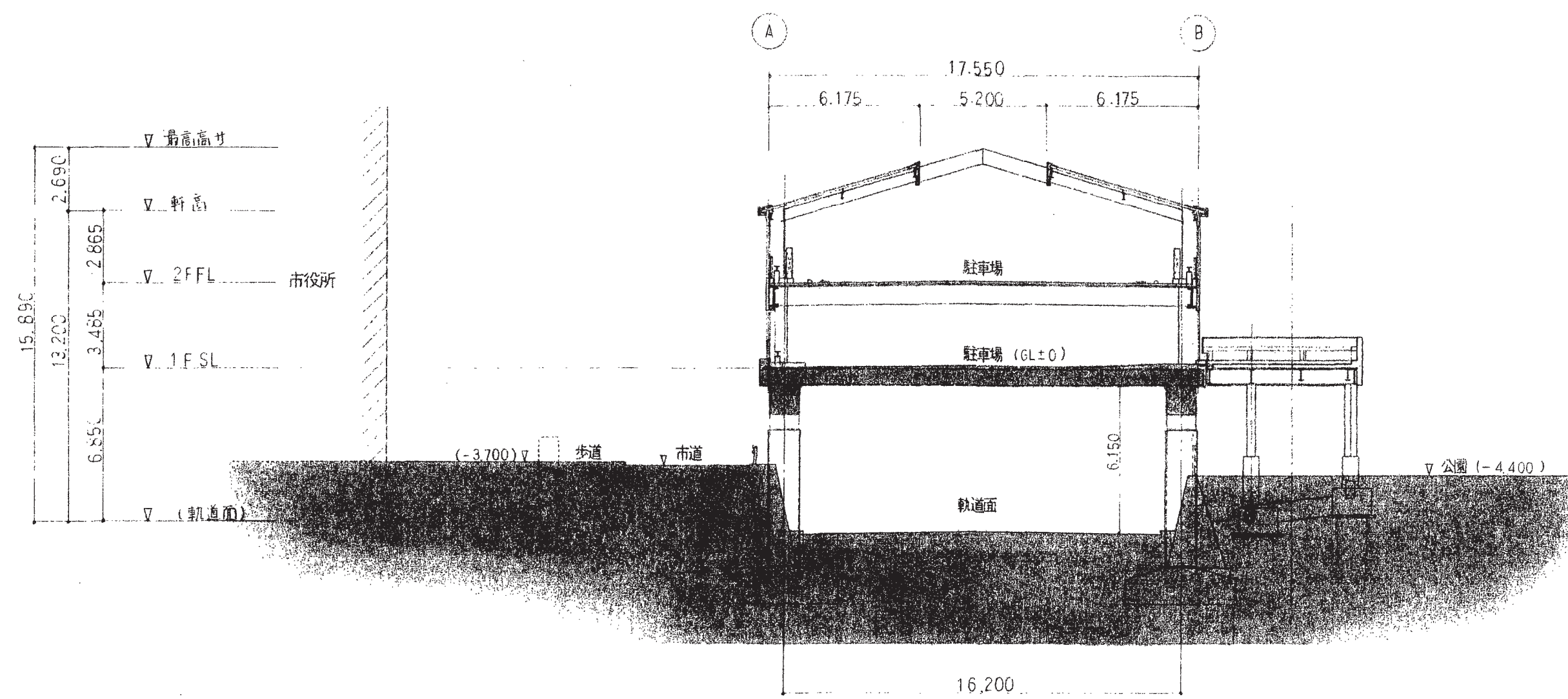
7通り 断面図 1:200
