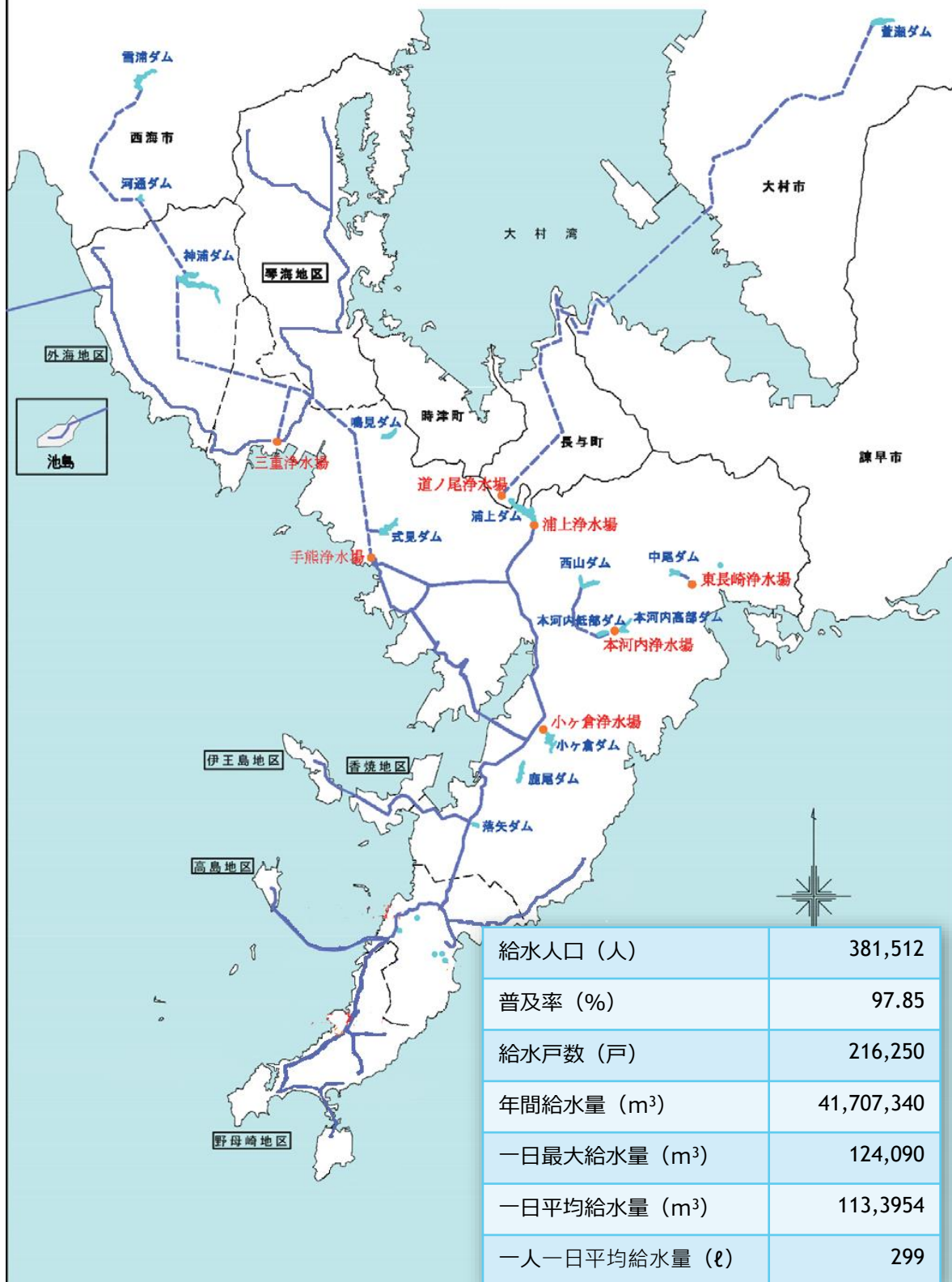
長崎市の主な水道施設及び令和５年度の給水状況
