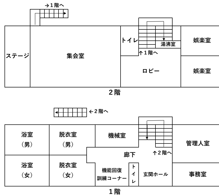
(イ) 平面図
