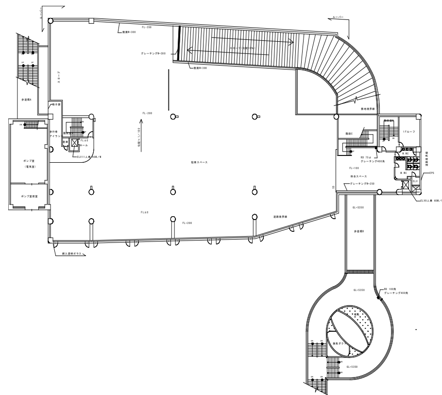
2階平面図
