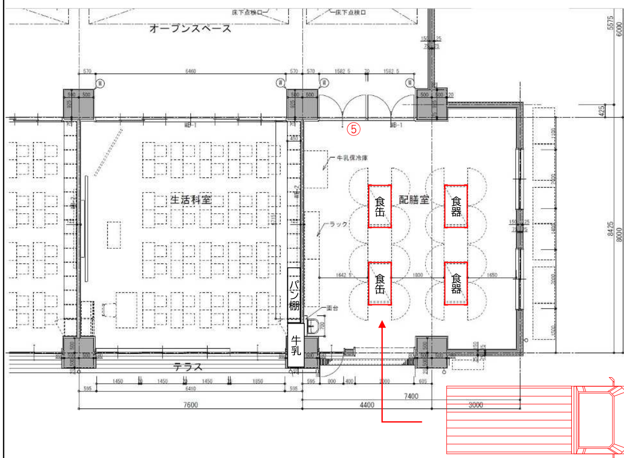
仁田佐古小学校コンテナ配置図
