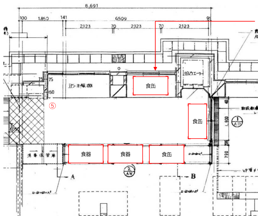
城山小学校 コンテナ配置図
