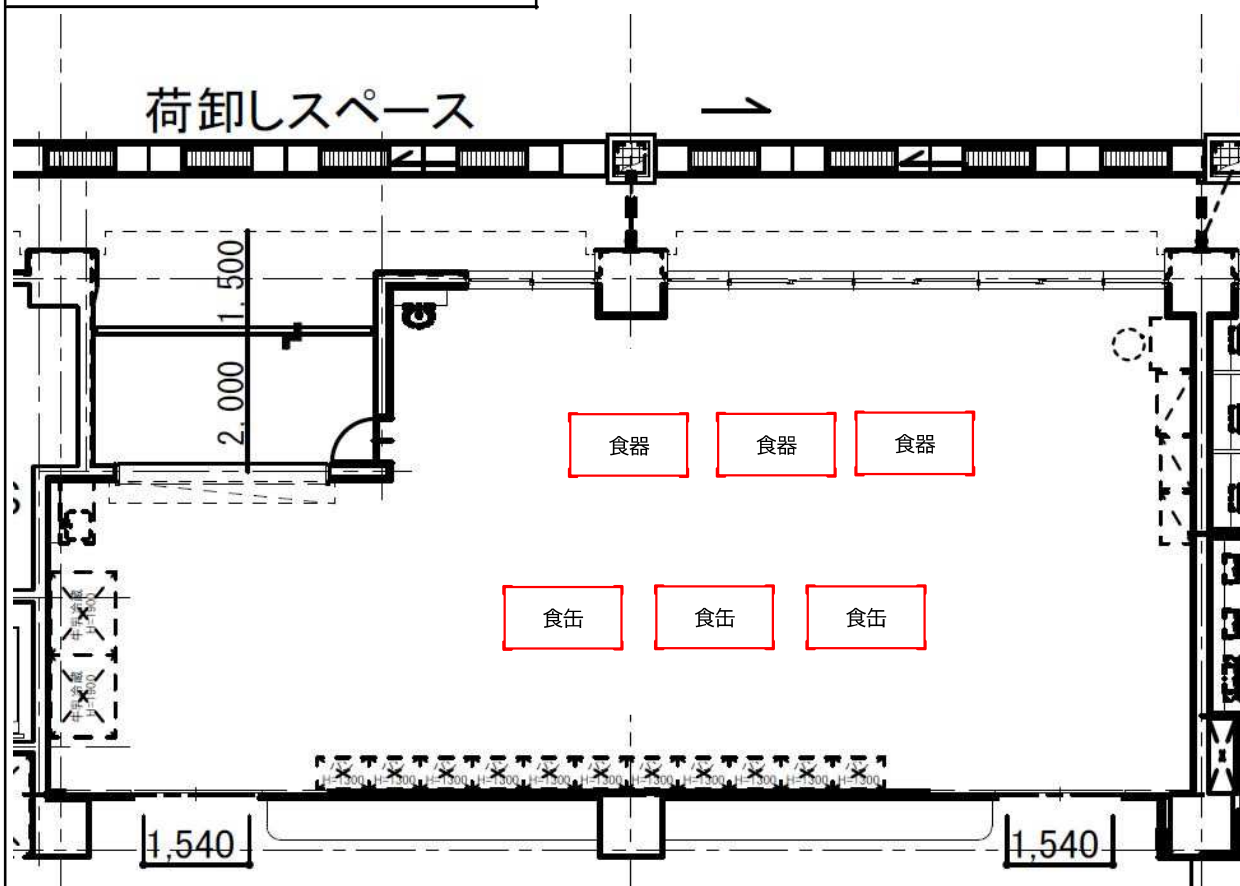
西浦上小学校 コンテナ配置図
