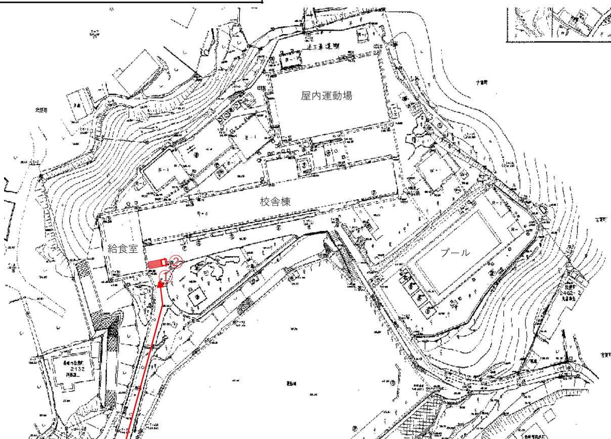
古賀小学校 配置図
