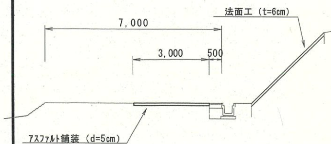
標準断面図
