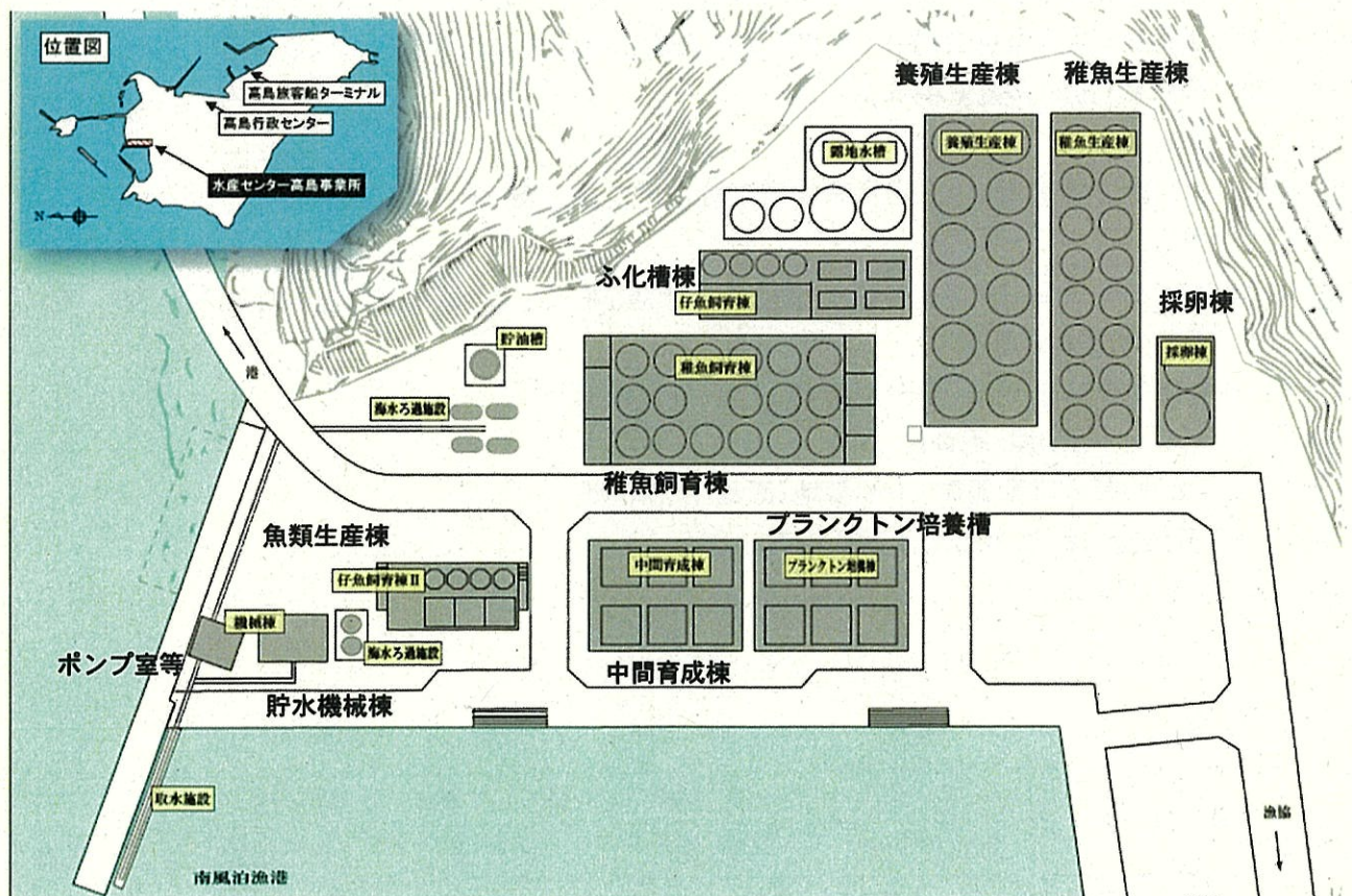
長崎市水産センター高島事業所の施設配置図
