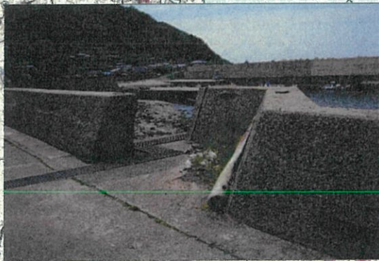
開口部対策 (例: 出津漁港)
