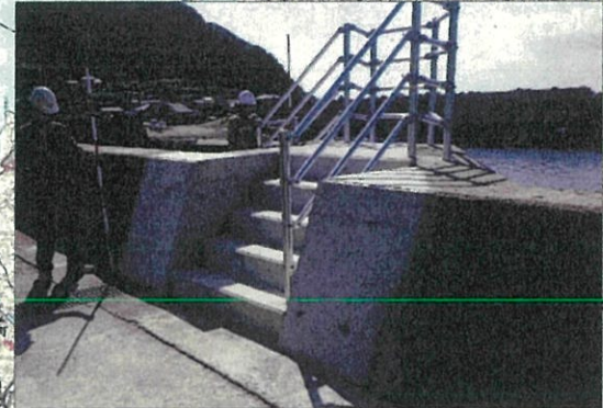
開口部対策 (例: 出津漁港)
