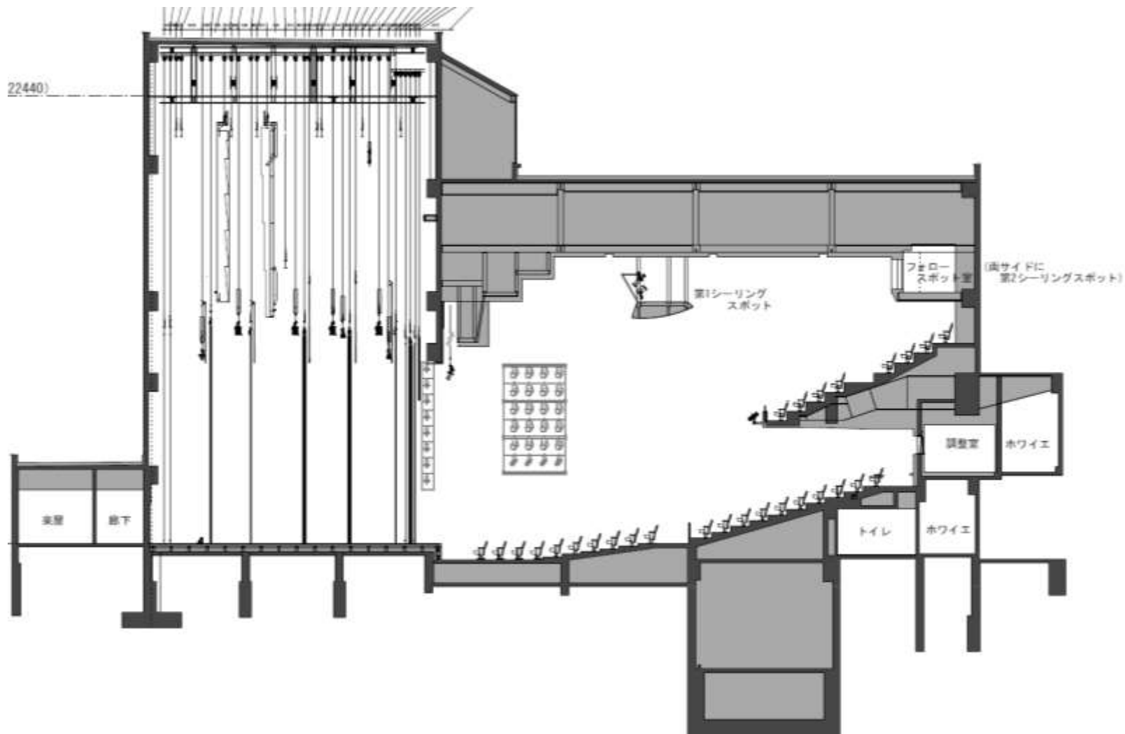
断面図
