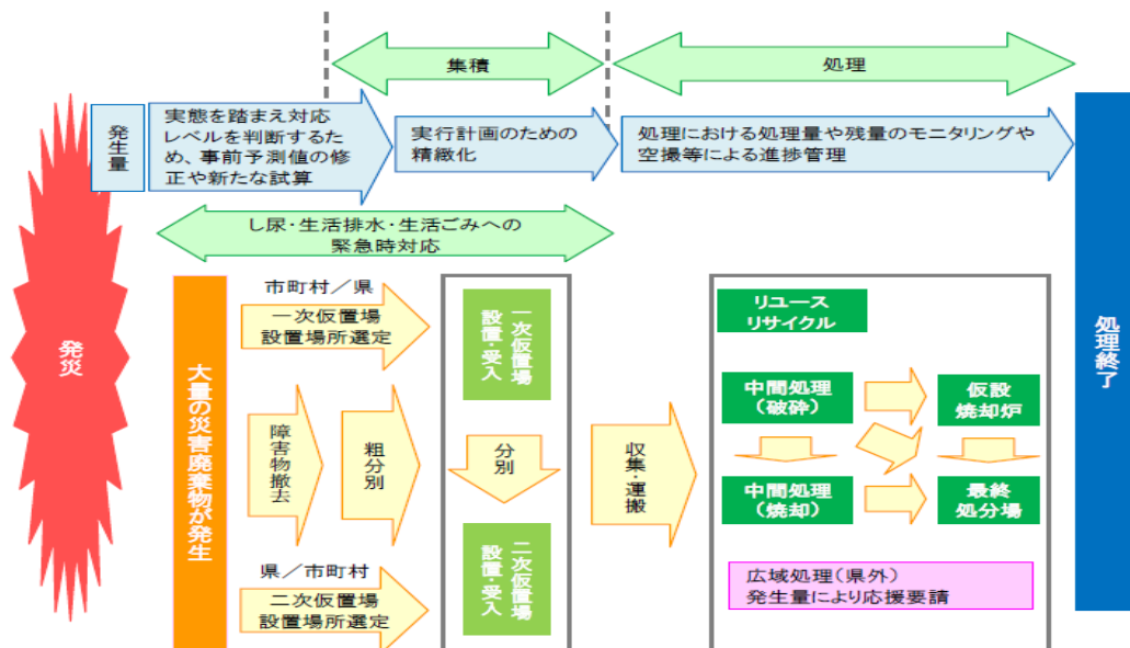
図 2-3-1 震災廃棄物処理の流れ
