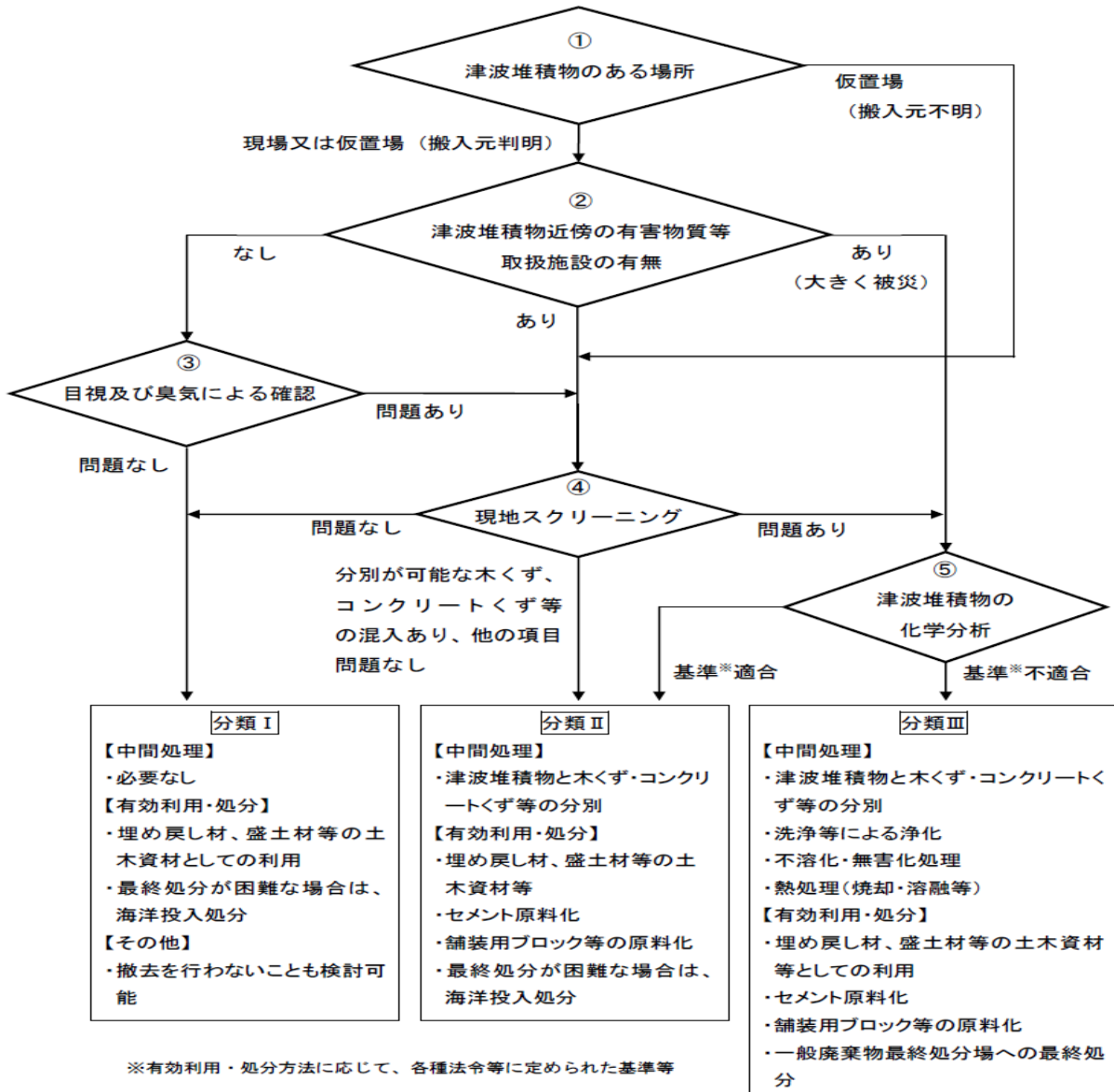
図2-3-7 津波堆積物の基本的処理フローチャート
