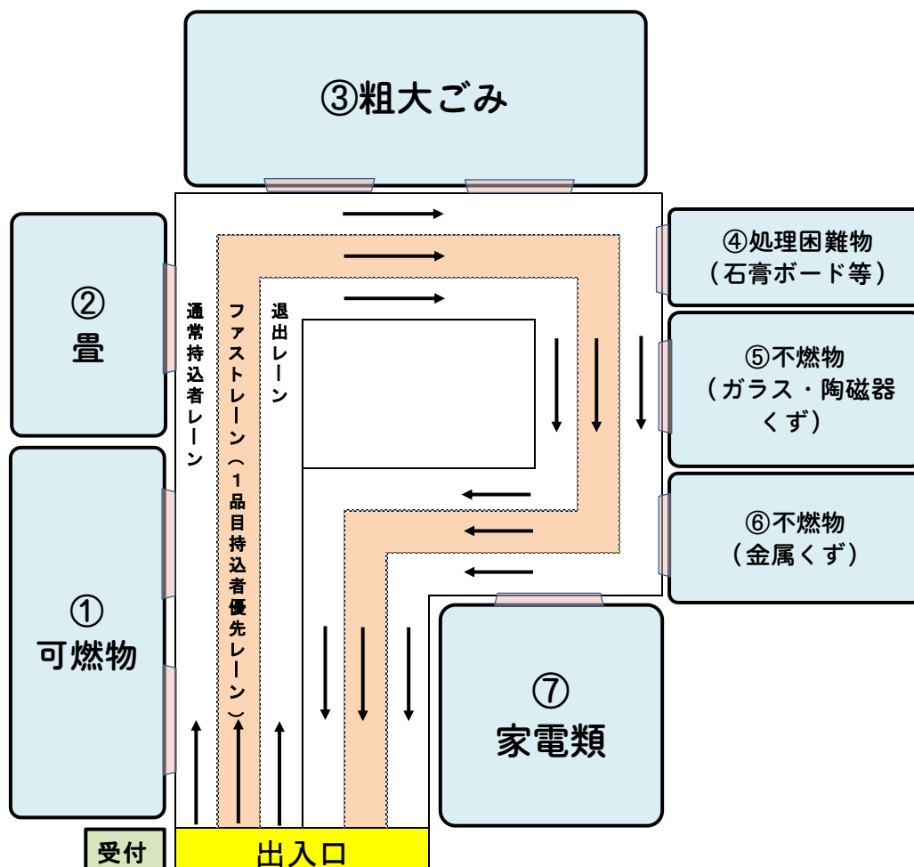
図 2-3-4 二次仮置場（中継仮置場）のレイアウトイメージ
