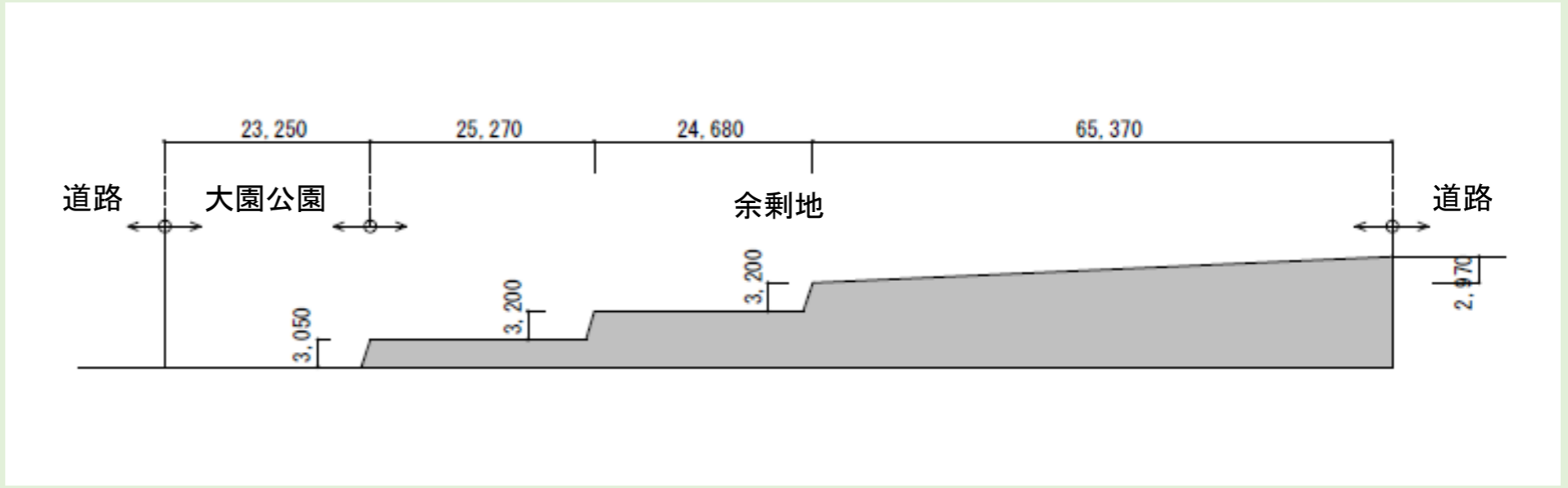
横断図
