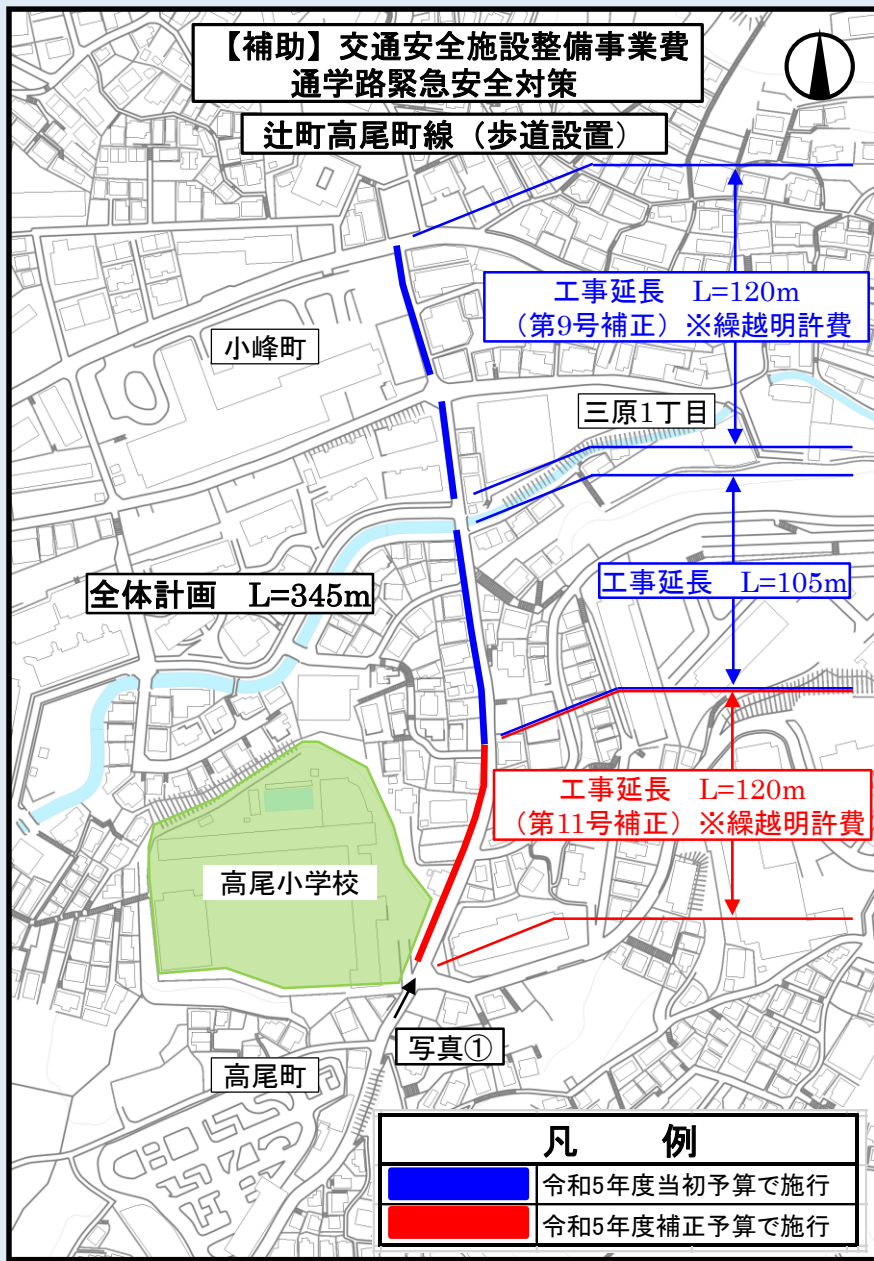
(1)位置図
