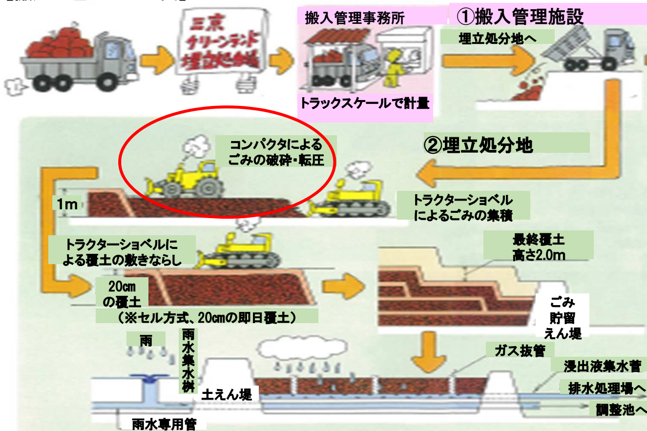
【搬入～埋立フロー図】
