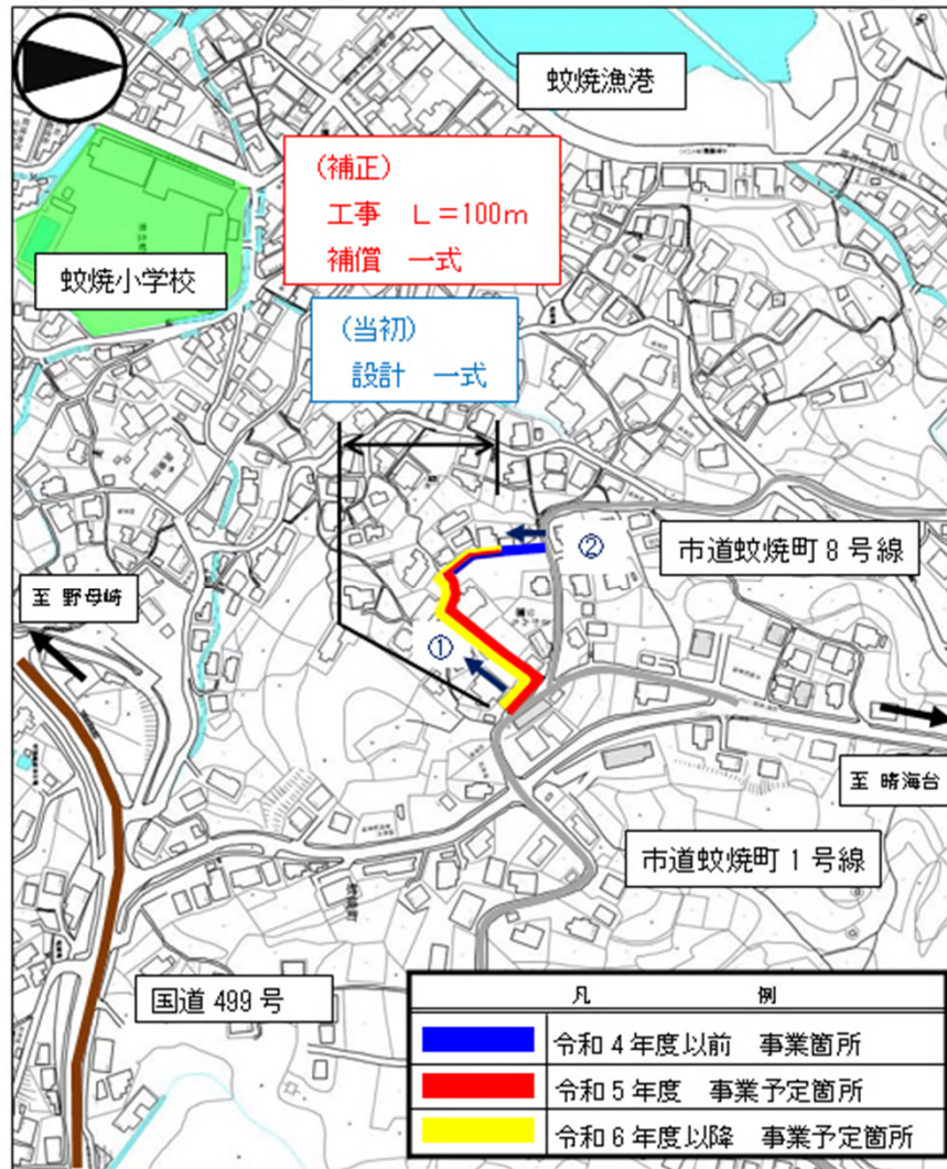
(1) 平面図
