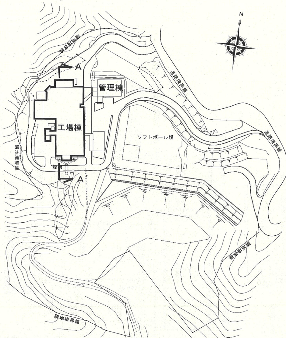
配置図
