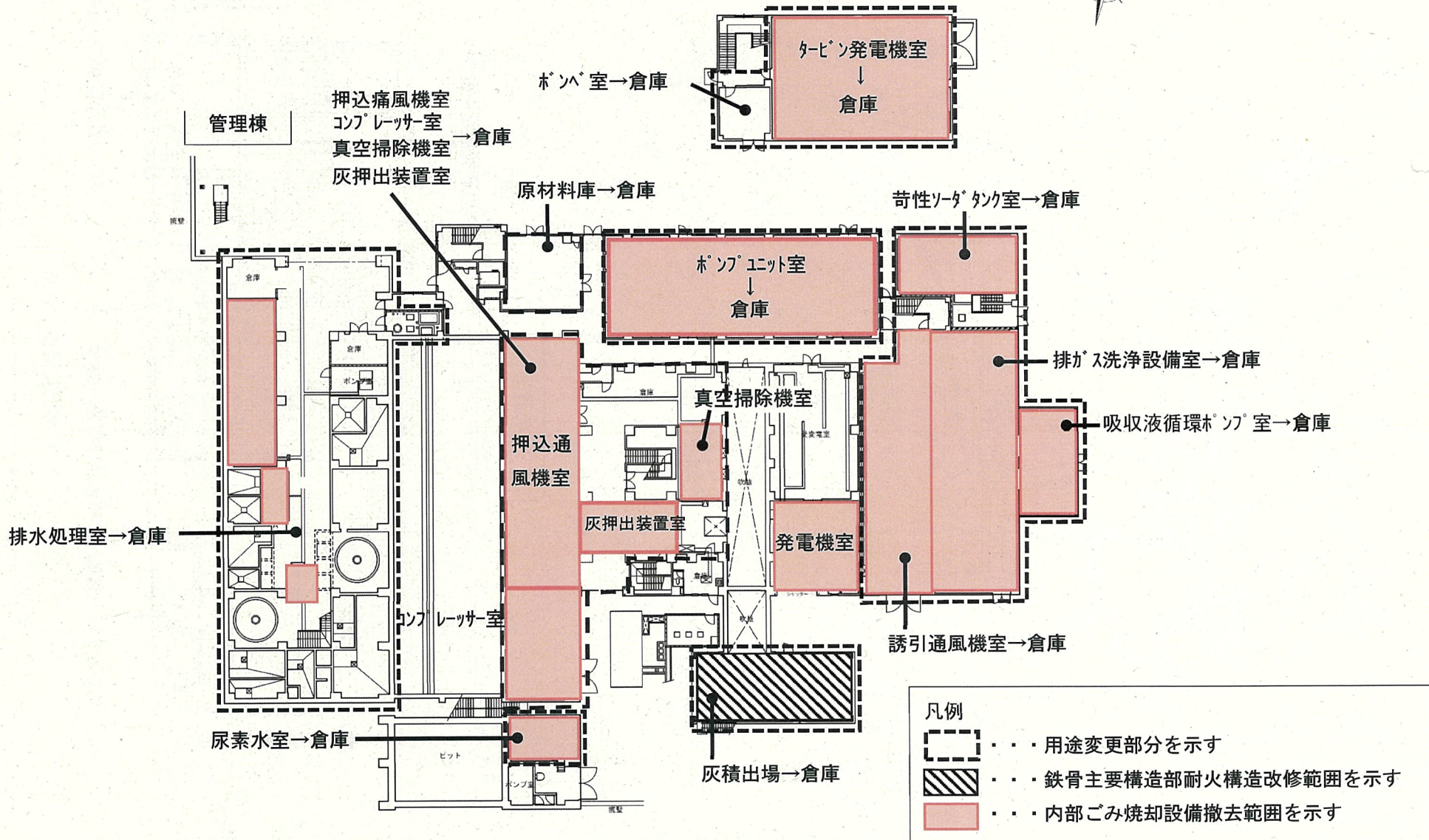
1階平面図
