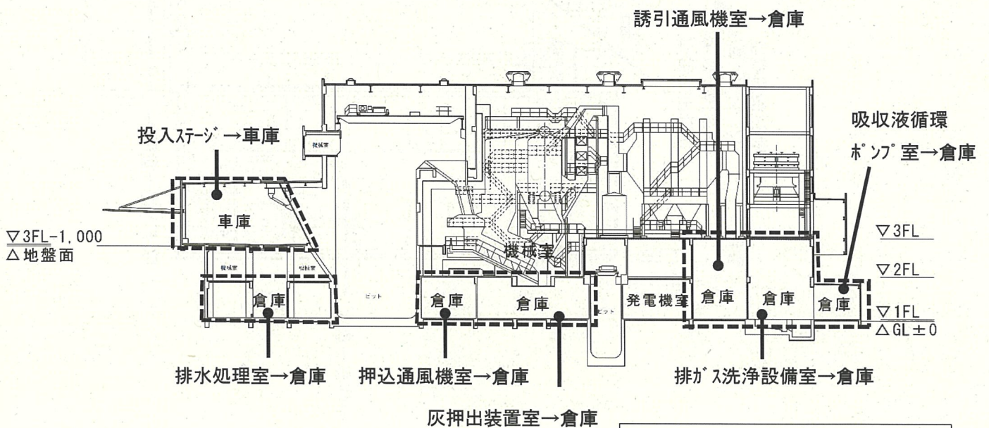
A-A' 断面図
