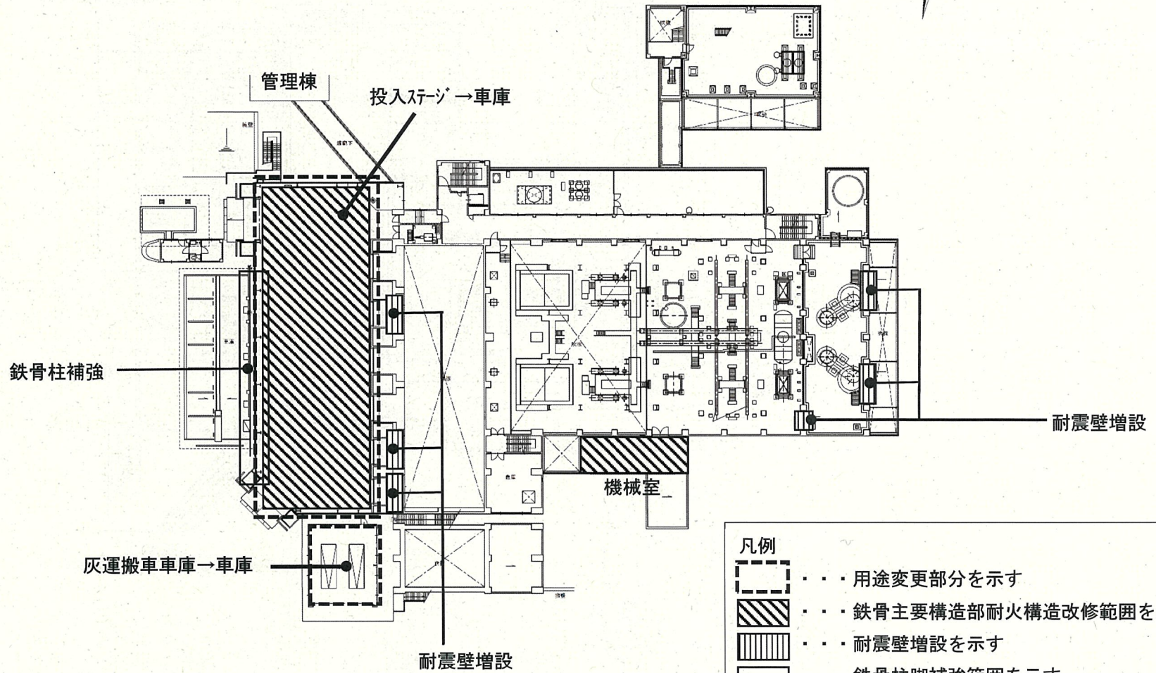
3階平面図
