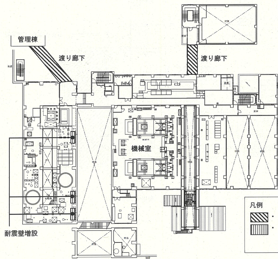
2階平面図
