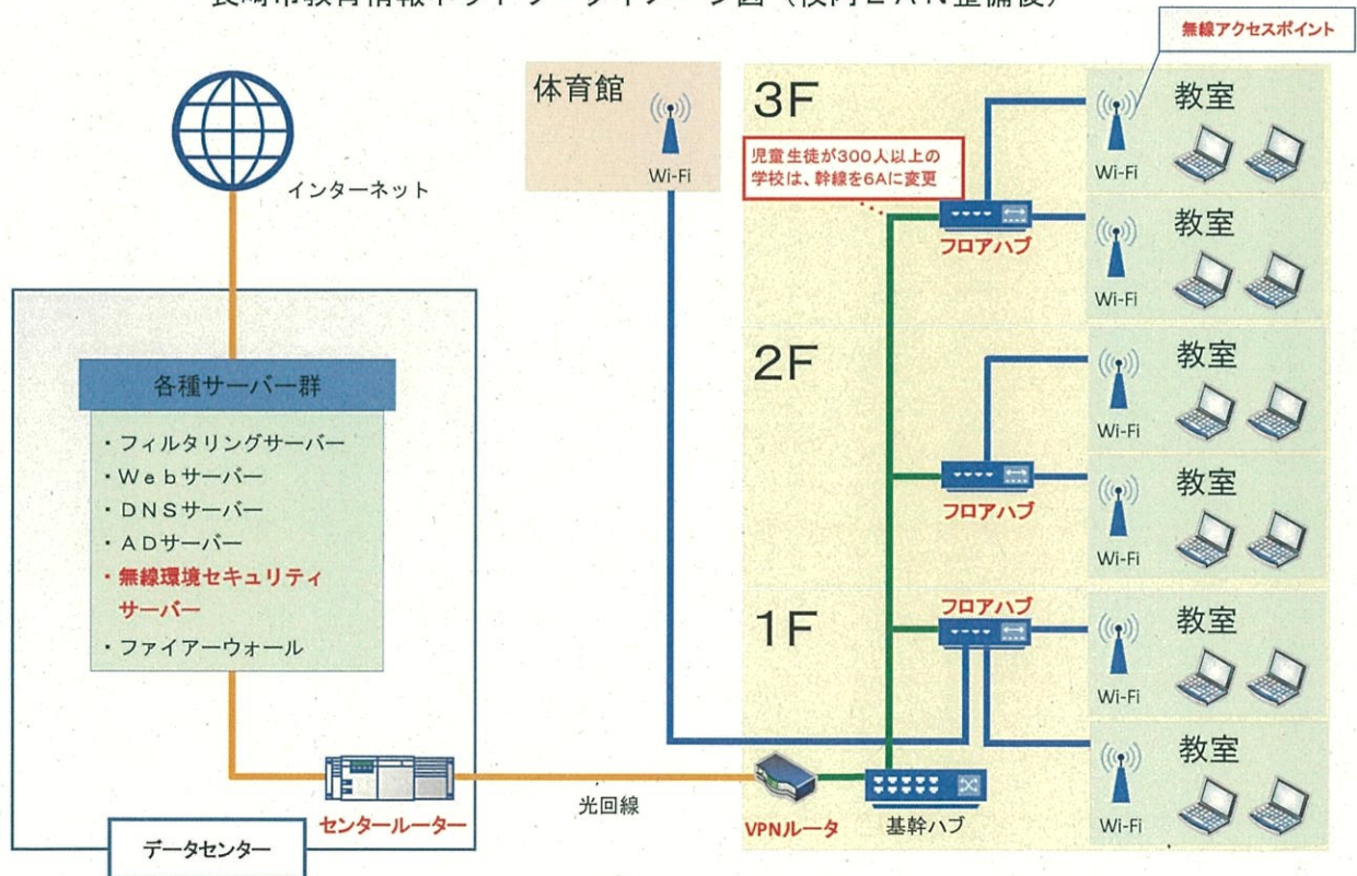
長崎市教育情報ネットワークイメージ図（校内LAN整備後）
