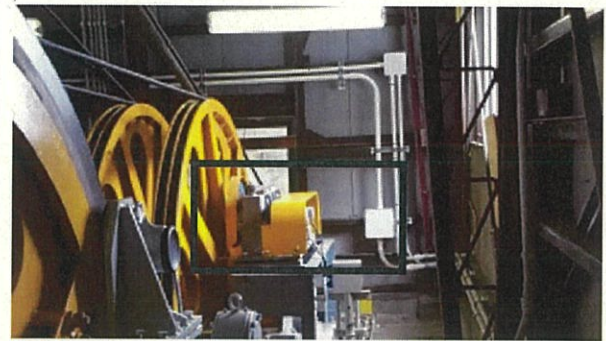
平衡索緊張重錘
