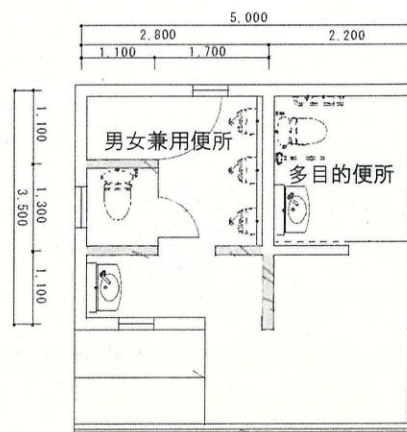
現況配置図
