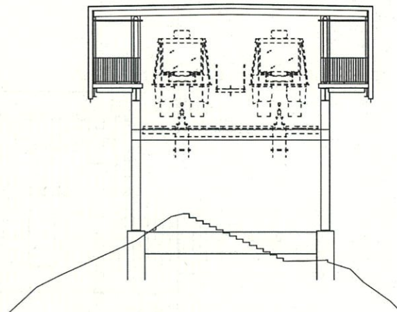
北立面図
