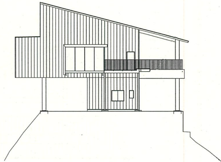
南立面図
