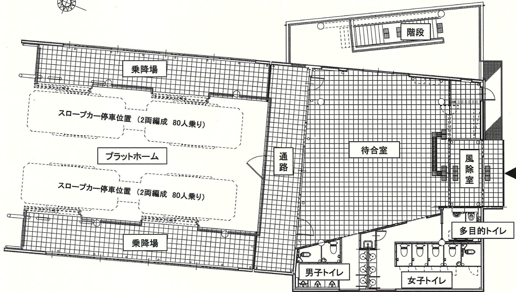
1 階 平 面 図
