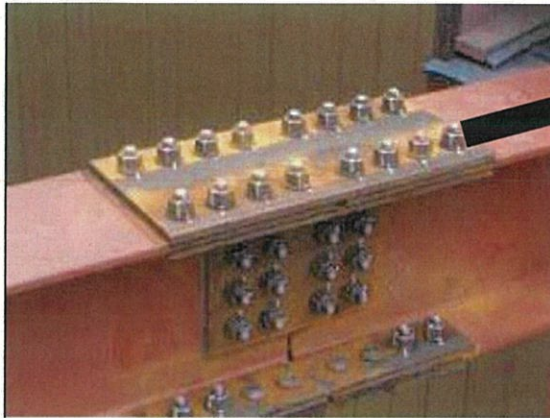
高力ボルトによる接合事例
