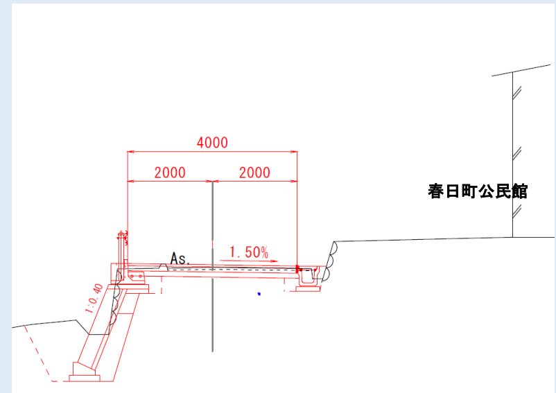
標準断面図
