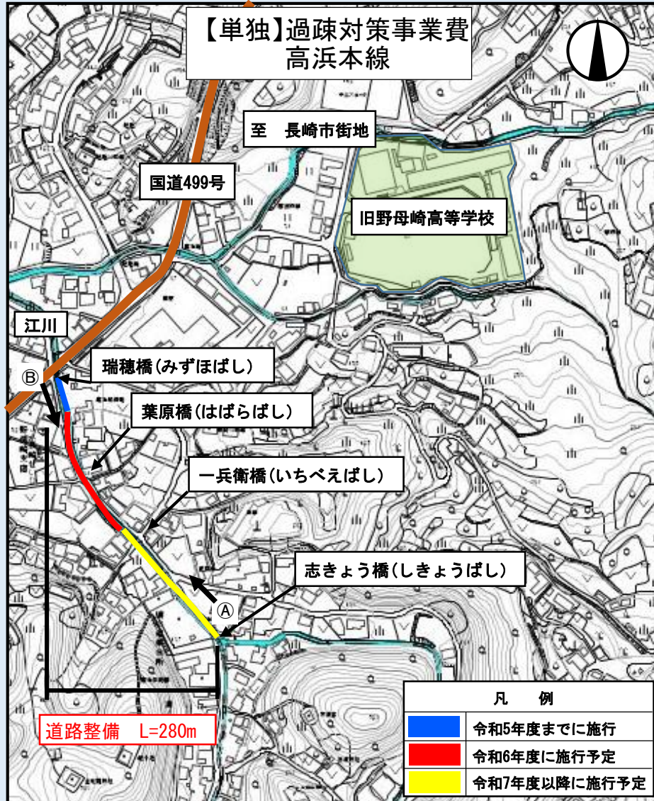
平面図
